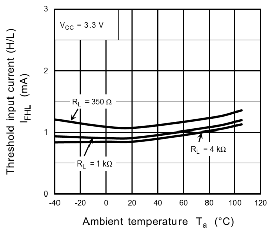
Fig. 11.2.9 I_{FHL} - T_a
