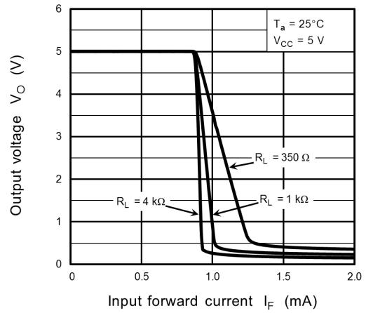
Fig. 11.2.8 V_O - I_F
