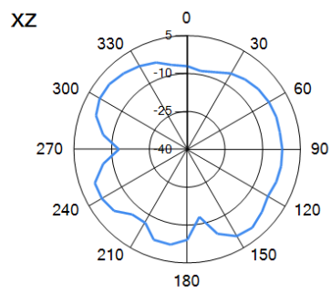
— 1.47GHz
