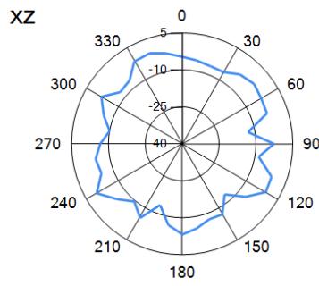
— 3.54GHz
