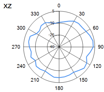
— 2.6GHz
